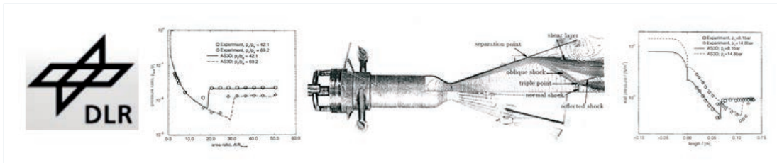
Separazione del flusso in un ugello di un razzo: la prima validazione del codice effettuata in collaborazione con DLR (German Aerospace Centrum).
