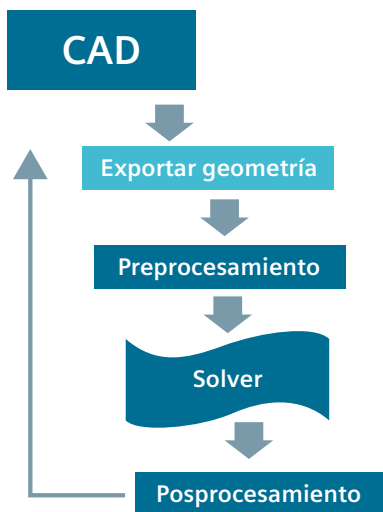
CFD tradicional: Proceso secuencial
