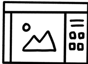
No-code
