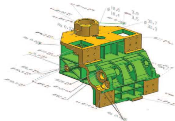
Abbildung 3: Dem NX CAD-Modell hinzugefügte PMI können verwendet werden, um die Feature-basierte Bearbeitung in NX CAM zu unterstützen.
