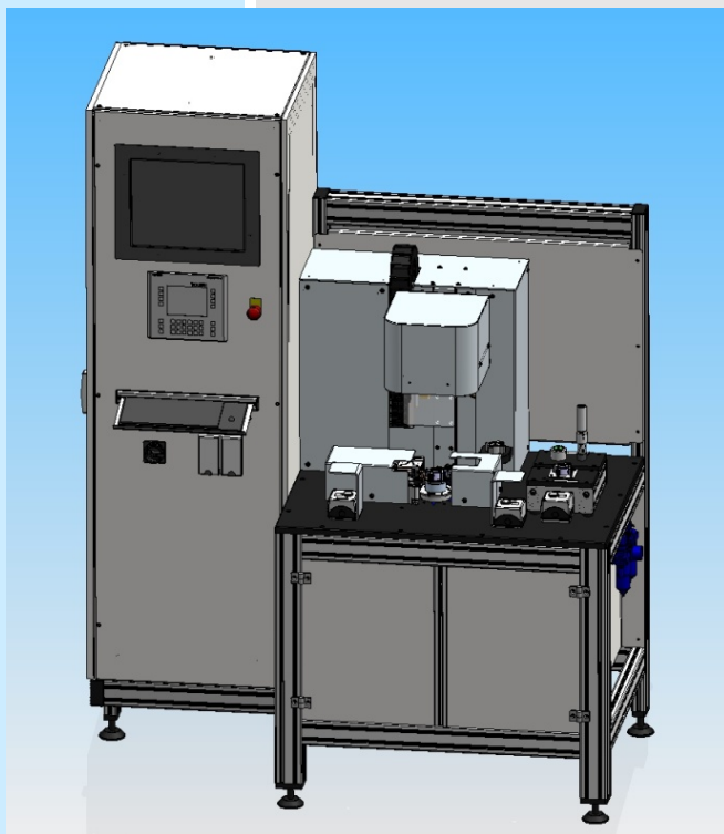
Das Bild zeigt: SPC Messplatz
