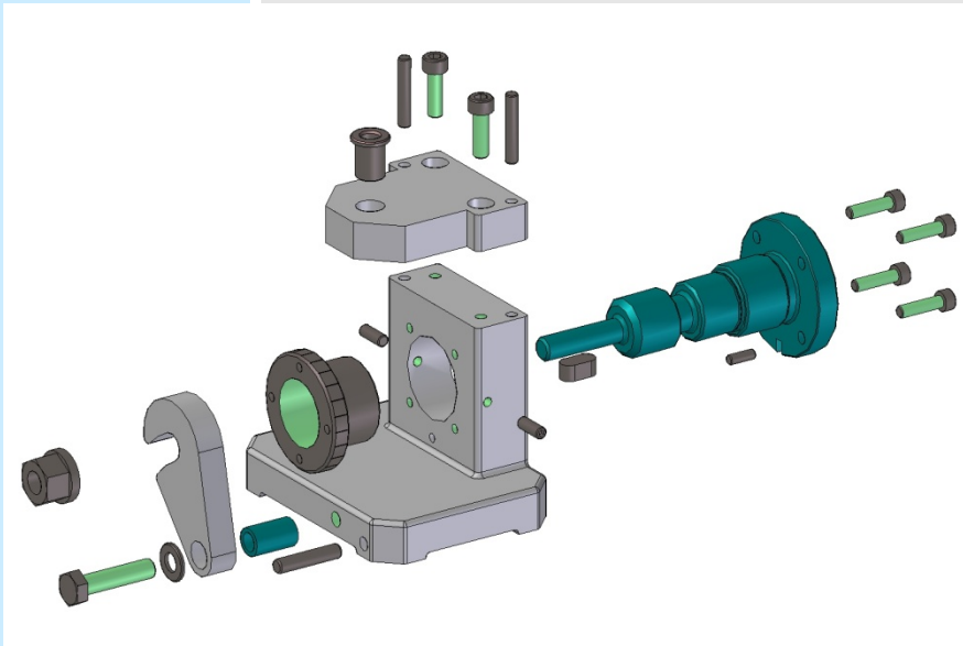
Das Bild zeigt: Bohrvorrichtung
